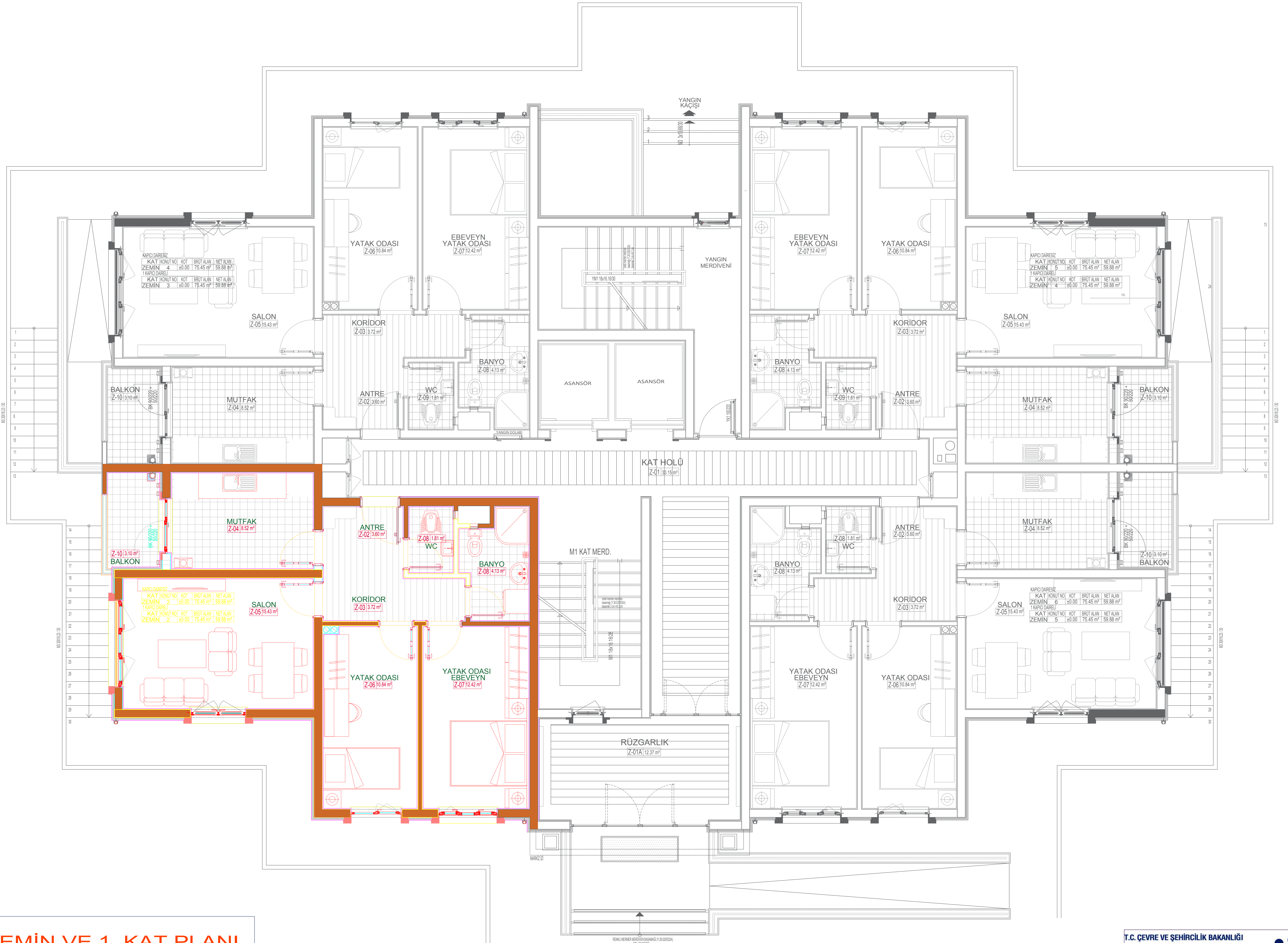
ZEMİN VE 1. KAT PLANI B5 TİPİ KONUT
